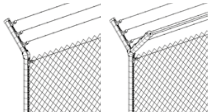
SUPLEMENTO BRAZO INCLINADO DOBLE CON ALAMBRE DE ESPINO (SOLO PARA TUBO LUX-80)
