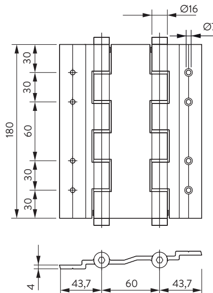
perfil R40
