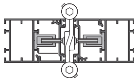
perfil R40
